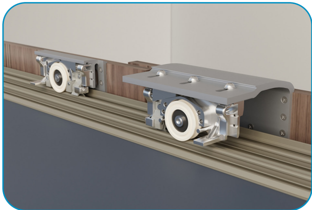
SISTEMAS DE CORRER SDS 800
