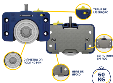
Roldana Sobreposta JP360
