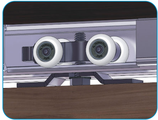
SISTEMA DE CORRER PANTOGRÁFICO
