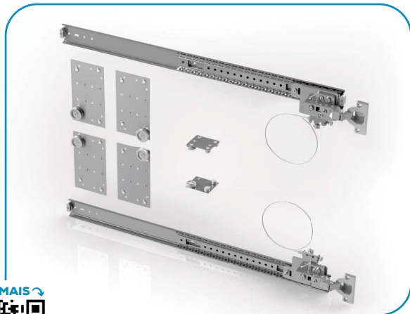
SISTEMA DE CORRER SOTELLO PARA PORTA DE EMBUTIR
