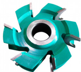
FRESA CABO DE VASSOURA
