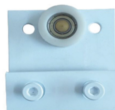
ROLDANA SIMPLES 2 Furos para Trilho 1030 Portas de até 30 kg
