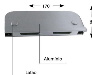
CONTRA FECHADURA PARA 1520MC
