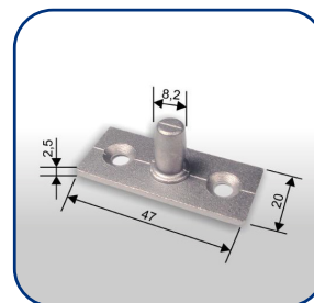
PIVÔ SUPERIOR
