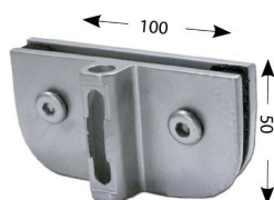
CONTRA TRINCO V/V SEM ABA PARA 1519
