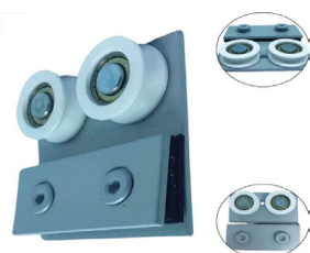
ROLDANA DUPLA PARA TRILHO 1030 PORTAS ATÉ 80 KG
